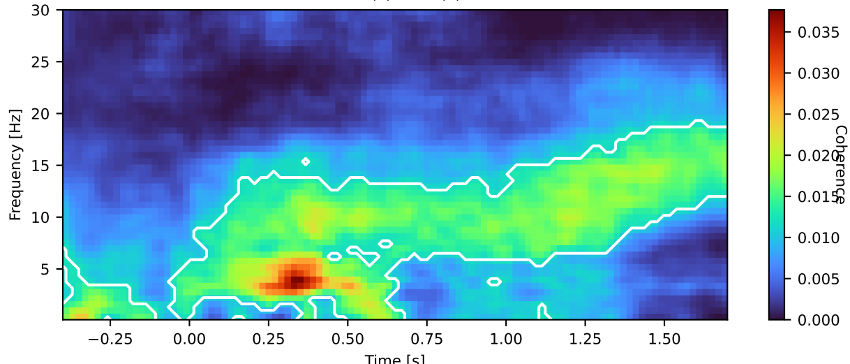
dPFC (6) - PEC (7)
